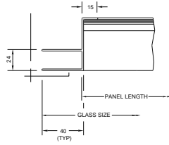
597. JAMB DETAIL
