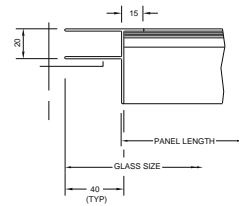
592. JAMB DETAIL
