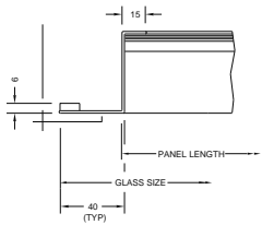
607. JAMB DETAIL
