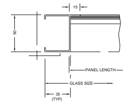
602. JAMB DETAIL
